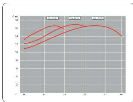
XF 100 elem.
