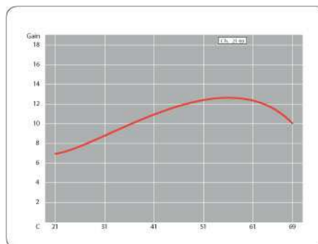
XF 32 elem.
