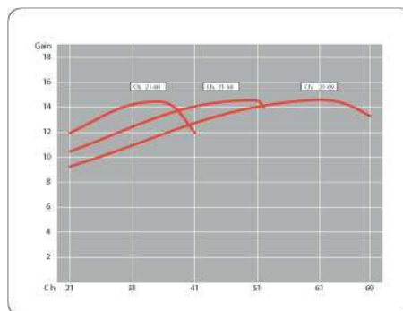
XF 52 elem.
